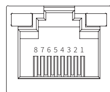
RJ45
